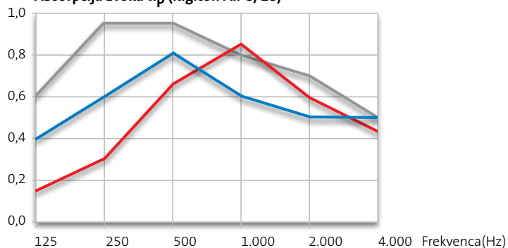
Absorpcija zvoka \alpha_p (Rigiton Air 8/18)
