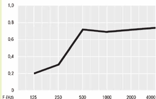
Stopnja absorpcije zvoka ( \alpha_S )
