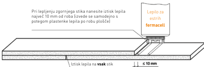
Slika 2: Drugi sloj plošč fermacell - iztisk lepila na rob plošče
