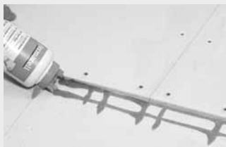
Lepilo na robu plošče 3. sloja proizvodov fermacell
