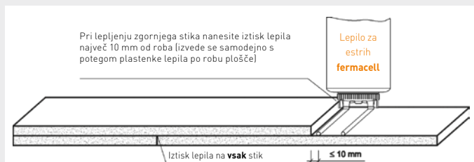
Slika 2: Drugi sloj plošč fermacell - iztisk lepila na rob plošče
