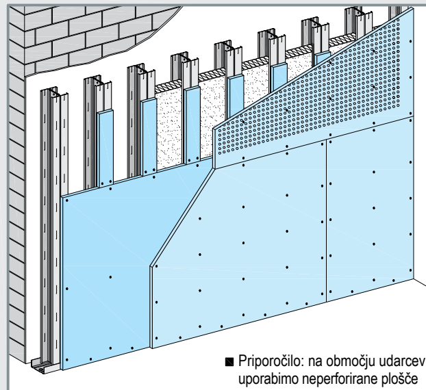
W623C-VO20 Stik s stropom - stropni C-profil
