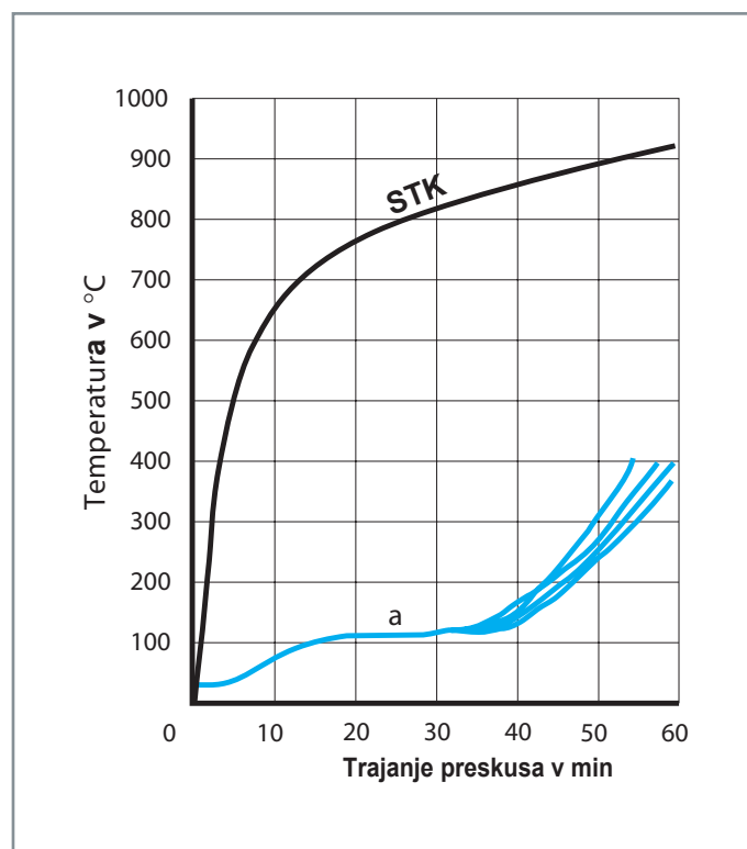
STK ... Standardna temperaturna krivulja požarne obremenitve
