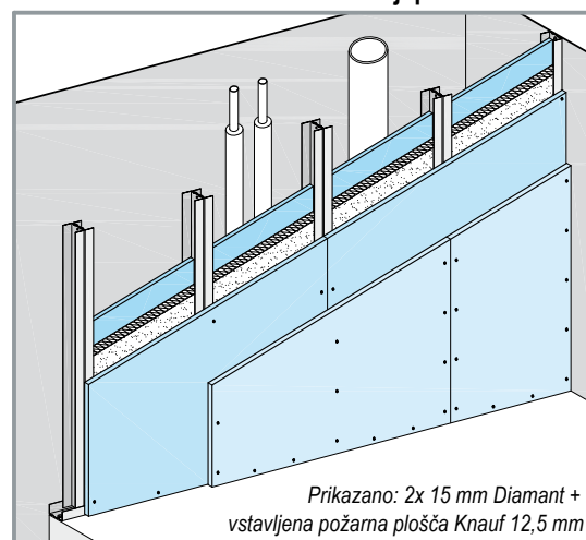
Verticalni prezezi
