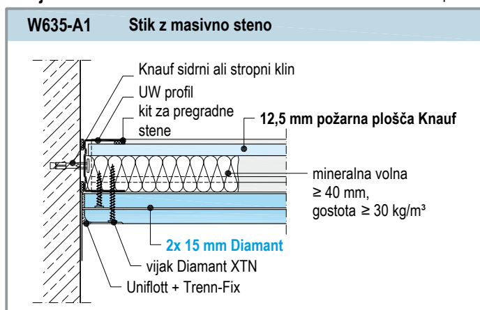
Horizontalni prerez
