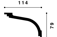
Z17 ARSTYL® 79 x 114 x 2000 mm
