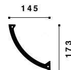
L3 ARSTYL® 173 x 145 x 2000 mm
