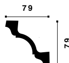
Z19 FLEX ARSTYL®
