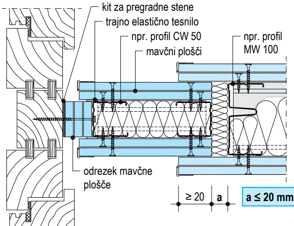
W112-A2 Drсни stik z leseno fasado
