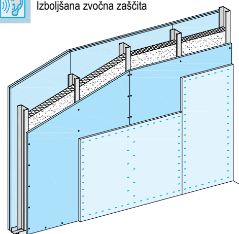
stik plošč - sredinska stojka
